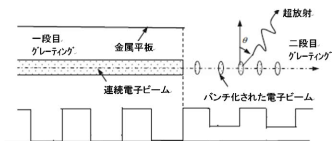
【図1】二段グレーティングスミス・パーセル放射機構
