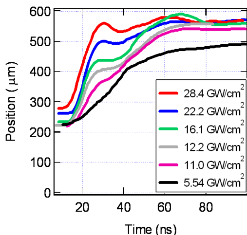
【図2】可視光計測により求められたプルームの先端位置の時間発展
