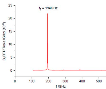
【図3】超放射スペクトル
