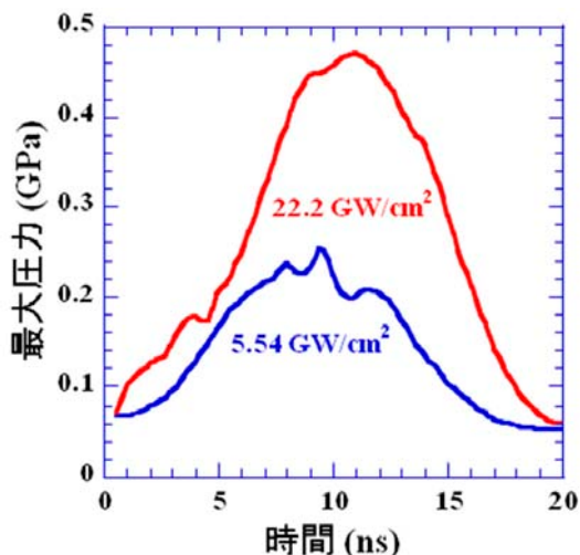
【図3】シミュレーションにより求めた、プルーム中の圧力の最大値の時間発展
