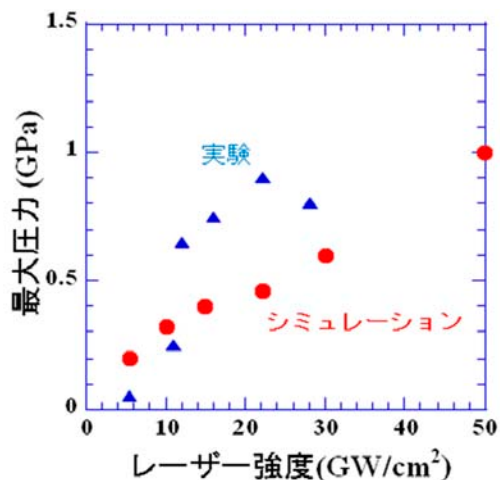
【図4】プルーム中の圧力の最大値の照射レーザー強度依存性
