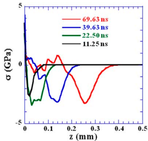
【図5】固体鉄中の応力分布の時間発展
