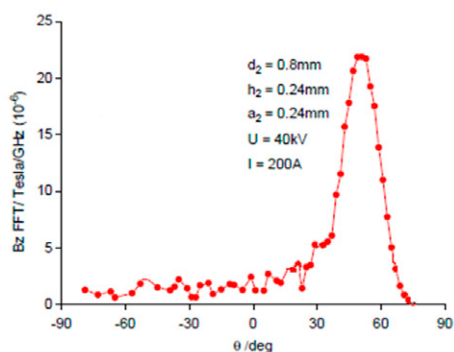
【図2】スミス・パーセル超放射空間分布
