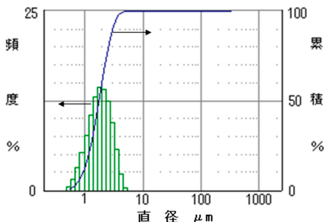
【図2】飛翔する鉛粒子の粒径頻度分布
